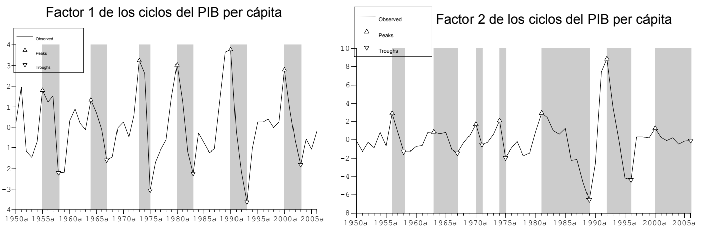
Figura 3: Ciclos comunes de Butterworth
