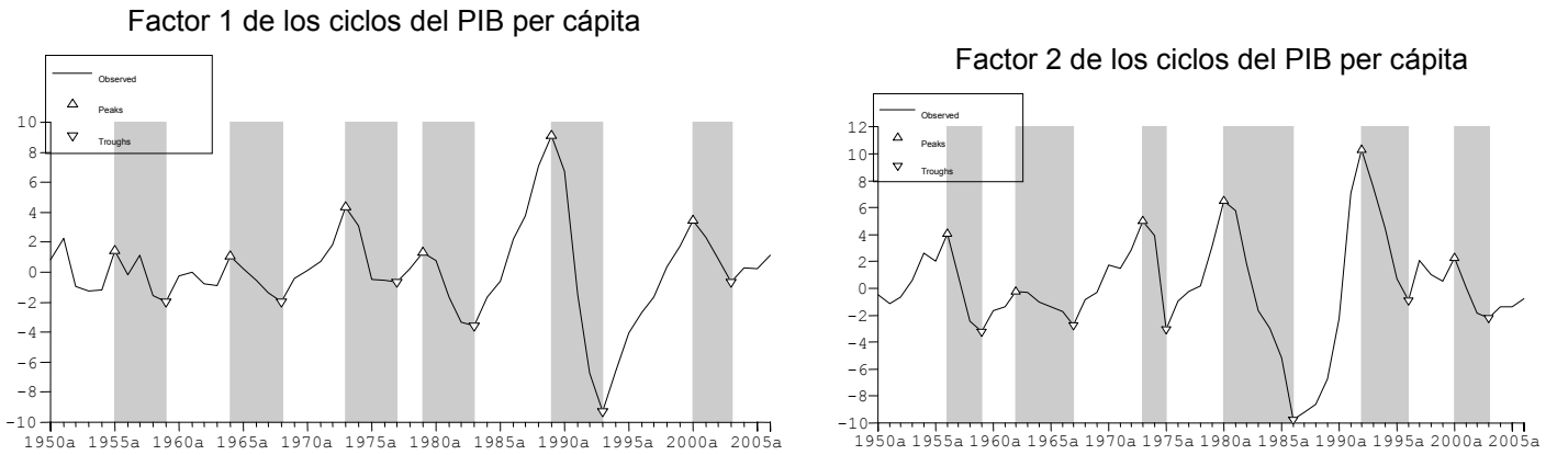
Figura 2: Ciclos comunes de Baxter-King .
