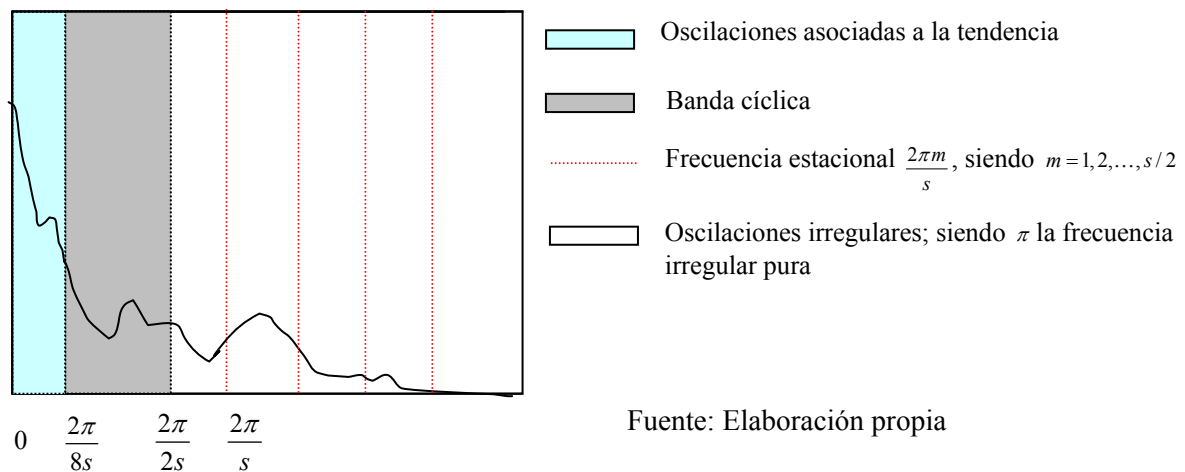
Figura 1: Espectro o función de densidad espectral de una serie temporal
