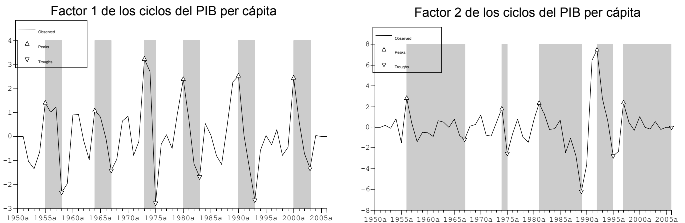
Figura 3: Ciclos comunes de Butterworth
