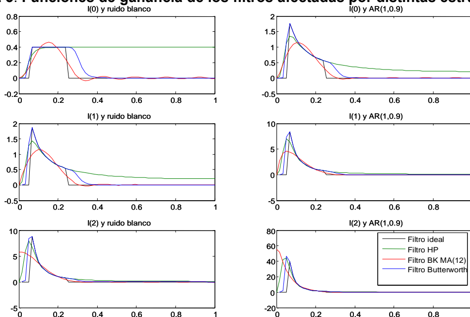
Figura 3: Funciones de ganancia de los filtros afectadas por distintas estructuras
