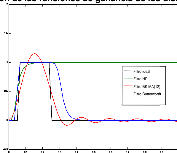
Figura 2: Comparación de las funciones de ganancia de los distintos filtros
